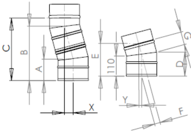
RÖRBÖJ 15°
