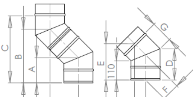
RÖRBÖJ 45°
