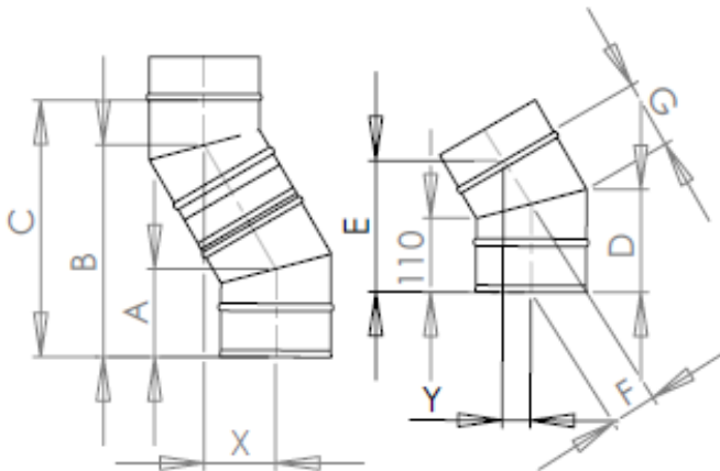
RÖRBÖJ 30°
